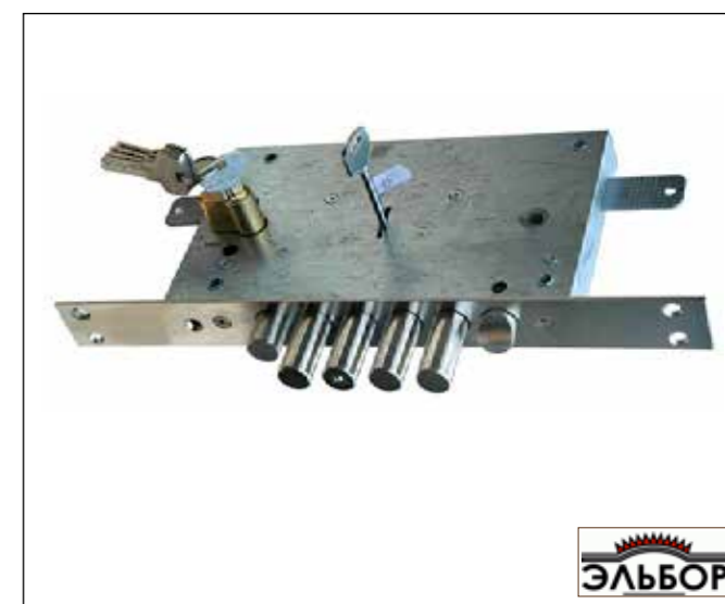
BORDER 3 ригеля с задвижкой
